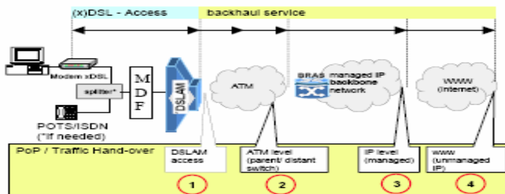
Figure 6.10 : Options des offres bitstream [Source : GRE]
