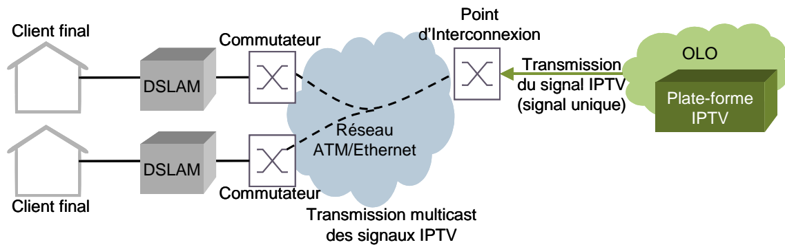
Figure 1: Description technique de la fonctionnalité multicast [Source : IBPT]
