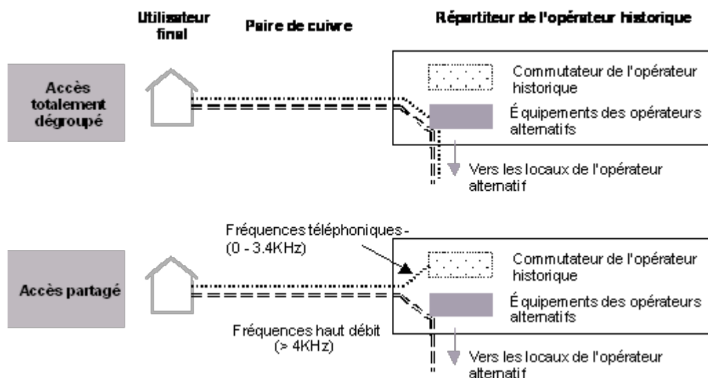
Figure 5.1 : Schéma du dégroupage total et du dégroupage partiel [Source : Analysys]
