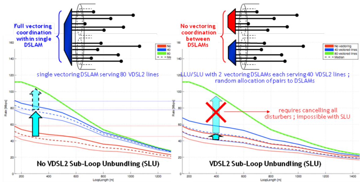
Figure 5.10 : impact du digital line management : sans dégroupage de sous-boucle locale (gauche) et avec dégroupage de sous-boucle locale (droite) (Bron : Alcatel-Lucent)
